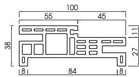
Đồ cửa 100 - PWF100 Door frame 100 - PWF100
