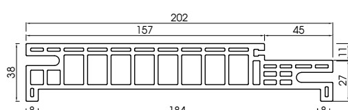
Đồ cửa 200 - PWF200 Door frame 200 - PWF200
