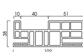
Đồ cửa 100H - PWF100H Door frame 100H - PWF100H
