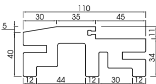
Đồ cửa 110 - PATB110 Door frame 110 - PATB110
