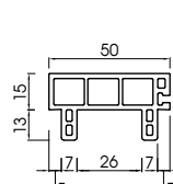
U đồ cửa 100H - PW 050 Door frame cap 100H - PW 050
