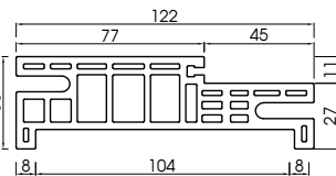
Đồ cửa 120 - PWF120 Door frame 120 - PWF120
