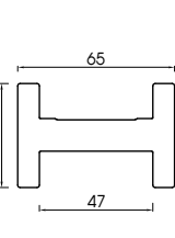
Thanh ray PABT 6543 Sliding door rail PABT 6543
