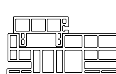
Bộ đồ cửa 100H Door frame set 100H
