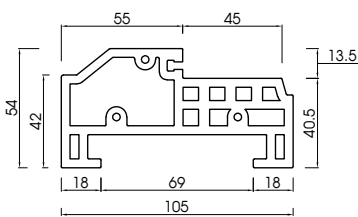
Đồ cửa 105 - PAK105 Door frame 105 - PAK105
