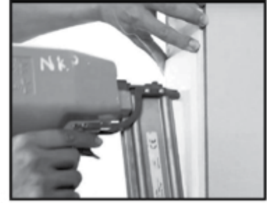
Bước 3: Bắn miếng bọt lên tường, sử dụng thước bắn laze, đảm bảo các miếng bọt được bắn thẳng hàng theo chiều đứng Step 3: Attach the pads into the wall with the laze ruler, make sure to attach the pads in a straight vertical line.
