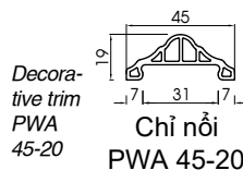
Decorative trim PWA 45-20 Chỉ nôi PWA 45-20 Nẹp kính PMK -G40 Glass frame PMK-G40
